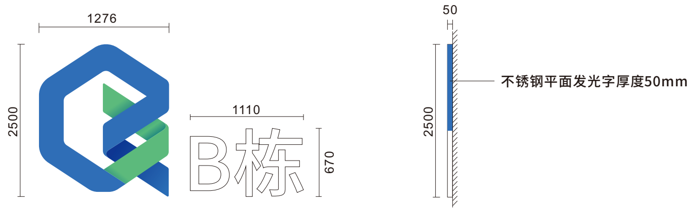
平面图
