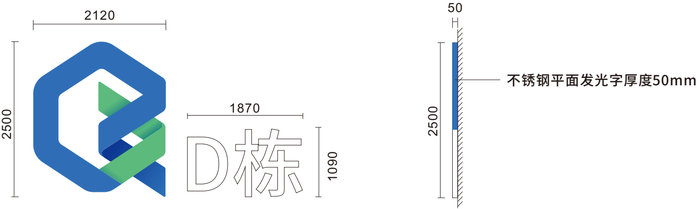
平面图
